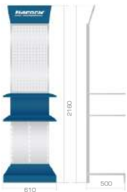
Стеллаж «Насосы плюс оборудование» узкий (2160/610/500)
