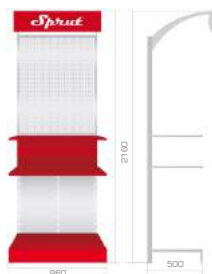
Стеллаж «Sprut» с лайт-боксом (2160/960/500)
