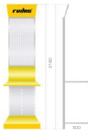
Стеллаж «Sprut» узкий (2160/610/500)
