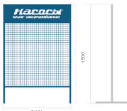
Стеллаж для фильтрационного оборудования, размеры 1000/1200
