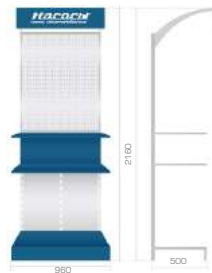
Стеллаж «Насосы плюс оборудование» с лайт-боксом (2160/960/500)
